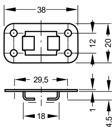
Guía de varilla
