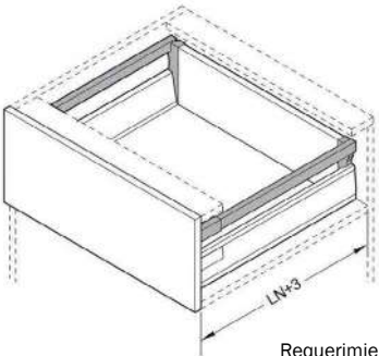
Requerimiento de espacio LN = Largo nominal
