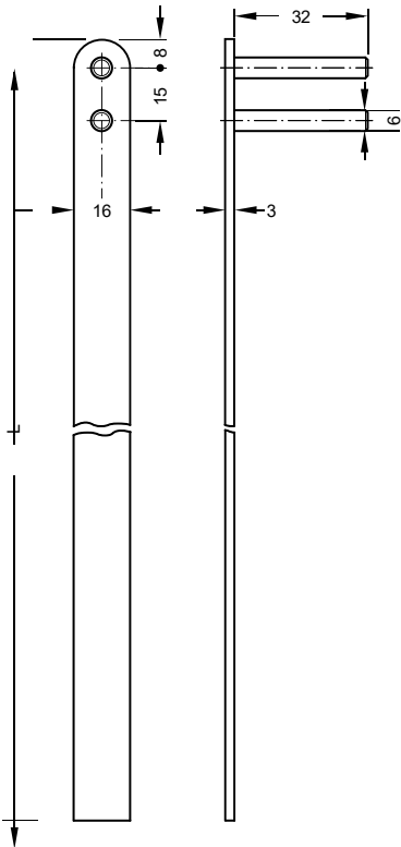
Varilla de cierre
