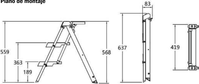
Plano de montaje
