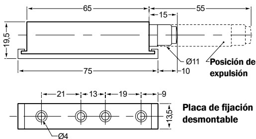
Plano de montaje
