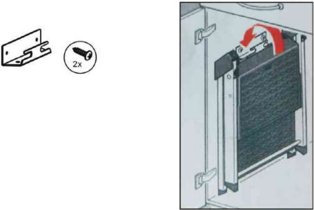
Soporte fijación lateral.
