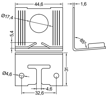
Escuadra para atornillar
