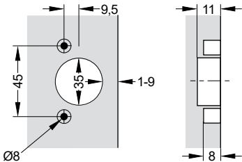
Tarugos para montaje rápido
