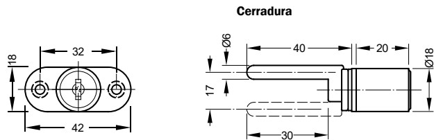
Plano de detalle
