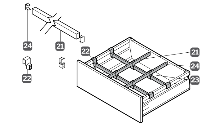
Accesorio divisor para ollero. Material: Plástico y aluminio.
