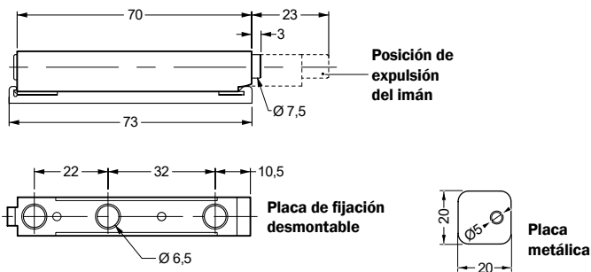
Plano de montaje
