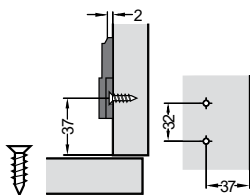
Plano de montaje
