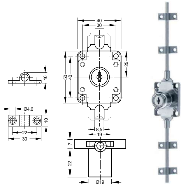
Plano de detalle
