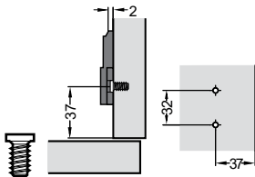
Plano de montaje
