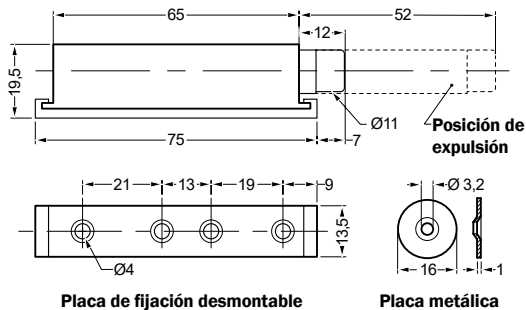
Plano de montaje
